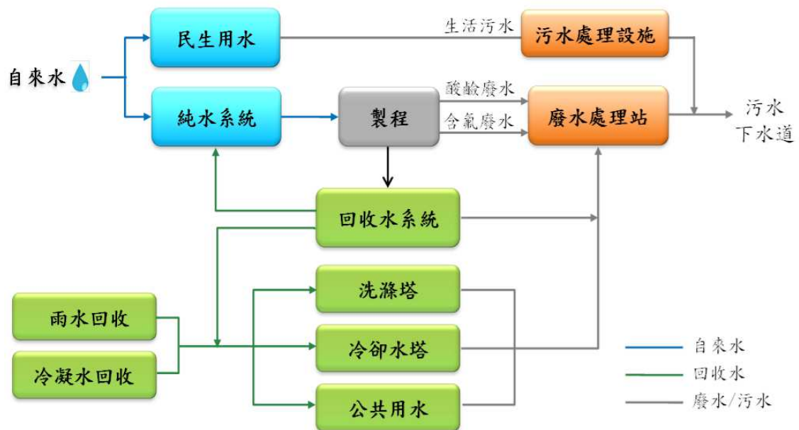
旺宏電子水資源循環使用示意圖
