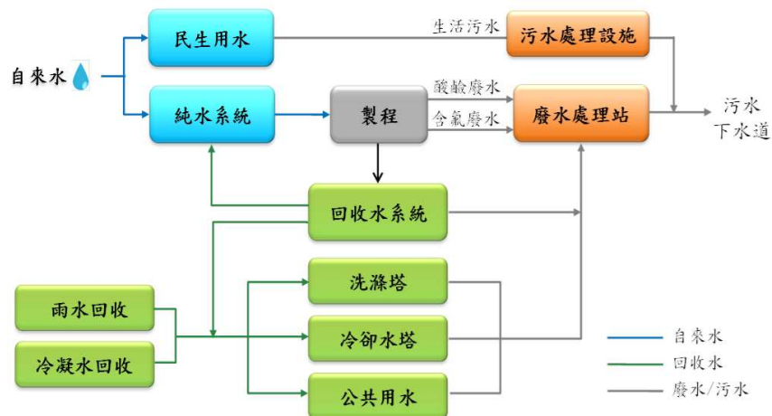
旺宏電子水資源循環使用示意圖
