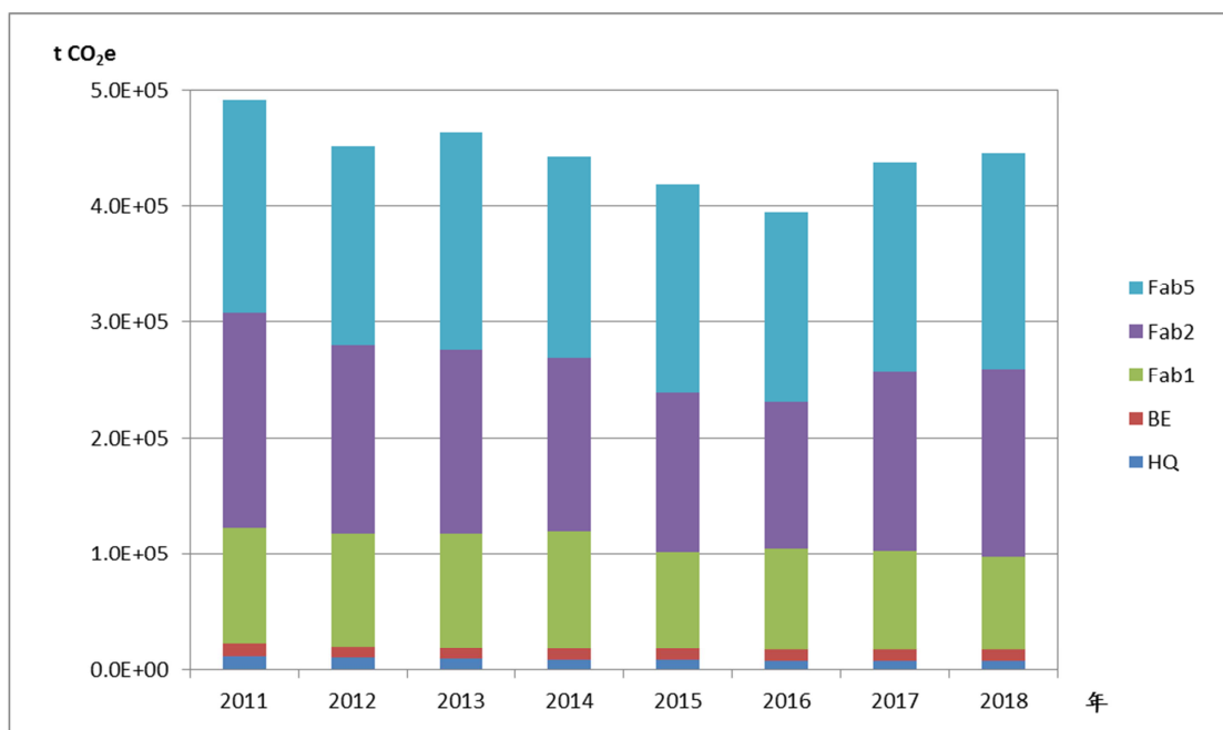
溫室氣體排放量趨勢圖
