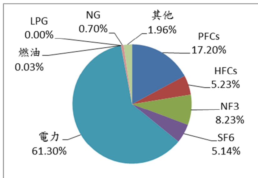
2018 年各種溫室氣體排放源占總排放量比例
