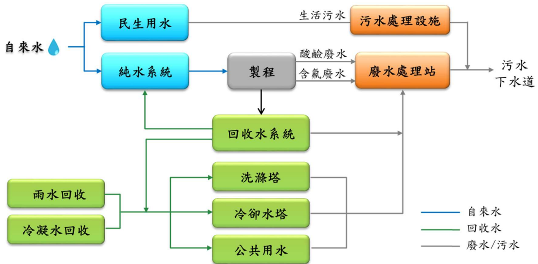
旺宏電子水資源循環使用示意圖
